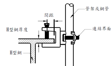
H型鋼及管架連結界面安裝圖
