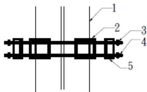
俯視圖
