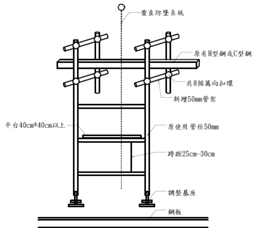
管架用調整基座及鋼板
