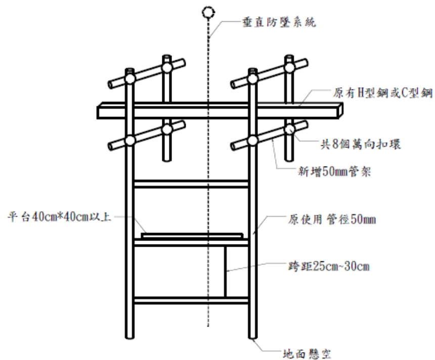
管架和H型鋼連結界面詳圖 (地面懸空)
