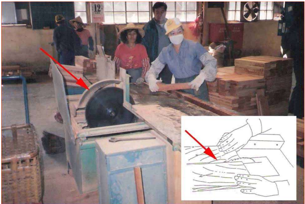
圓盤鋸安全裝置- 撐縫片
