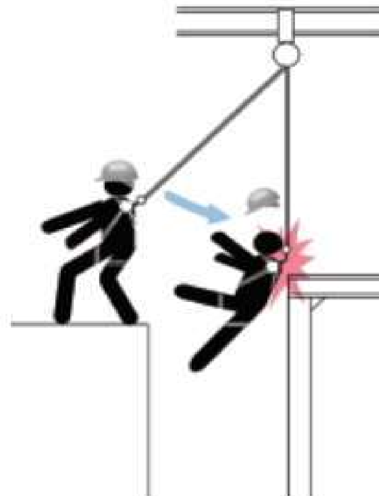
圖2 鐘擺效應
