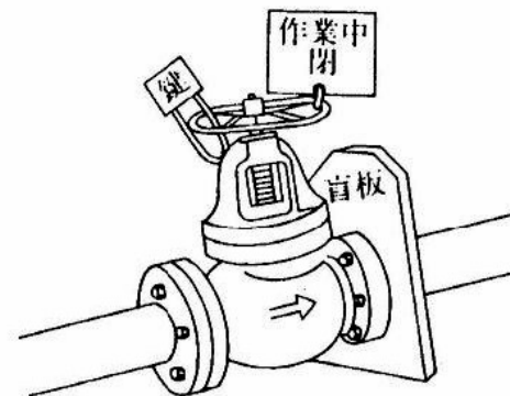
圖 4.3 爲了完全關緊閥而使用的盲板
