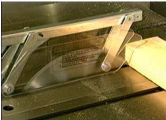
刃部接觸預防裝置
