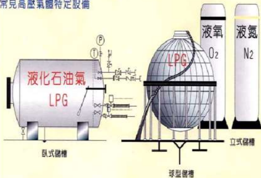
常見高壓氣體特定設備
